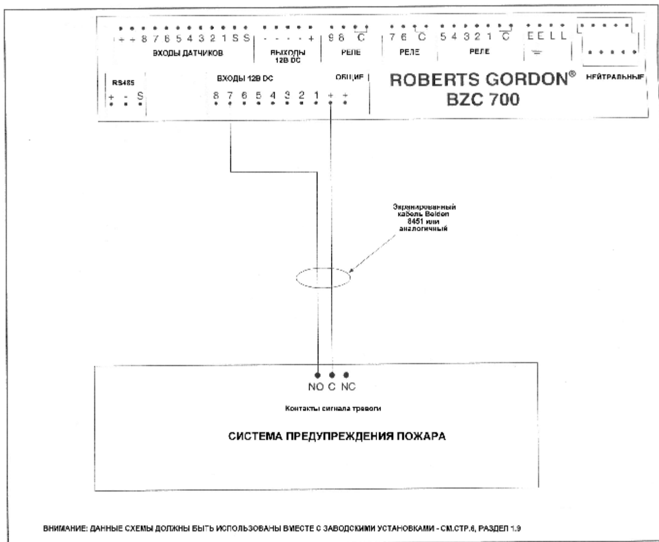
РИСУНОК 21 Монтажная схема отключения по пожарной безопасности
