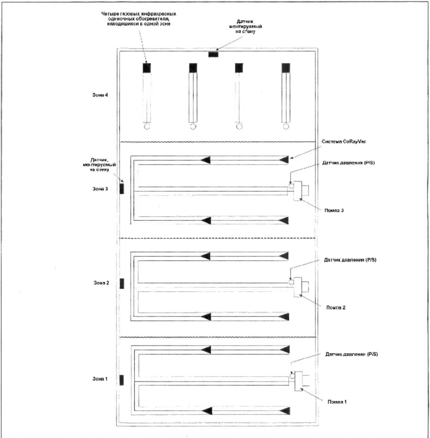
РИСУНОК 1 Пример чертежа расположения оборудования
