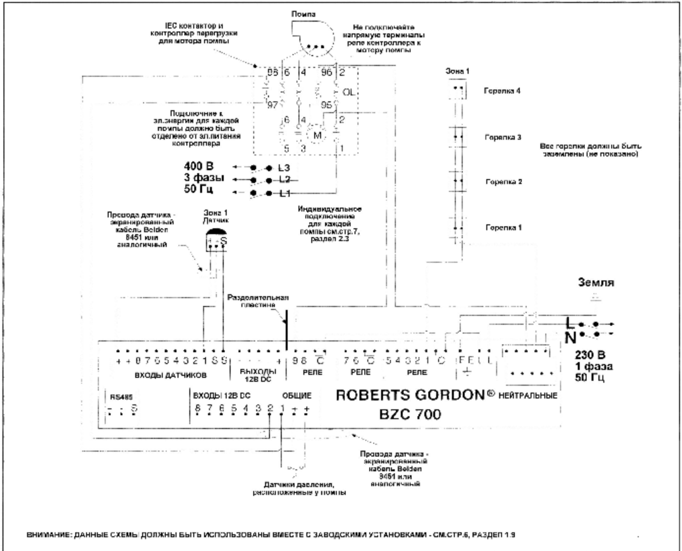
РИСУНОК 17 Типичная монтажная схема отображения отключения трехфазной помпы
