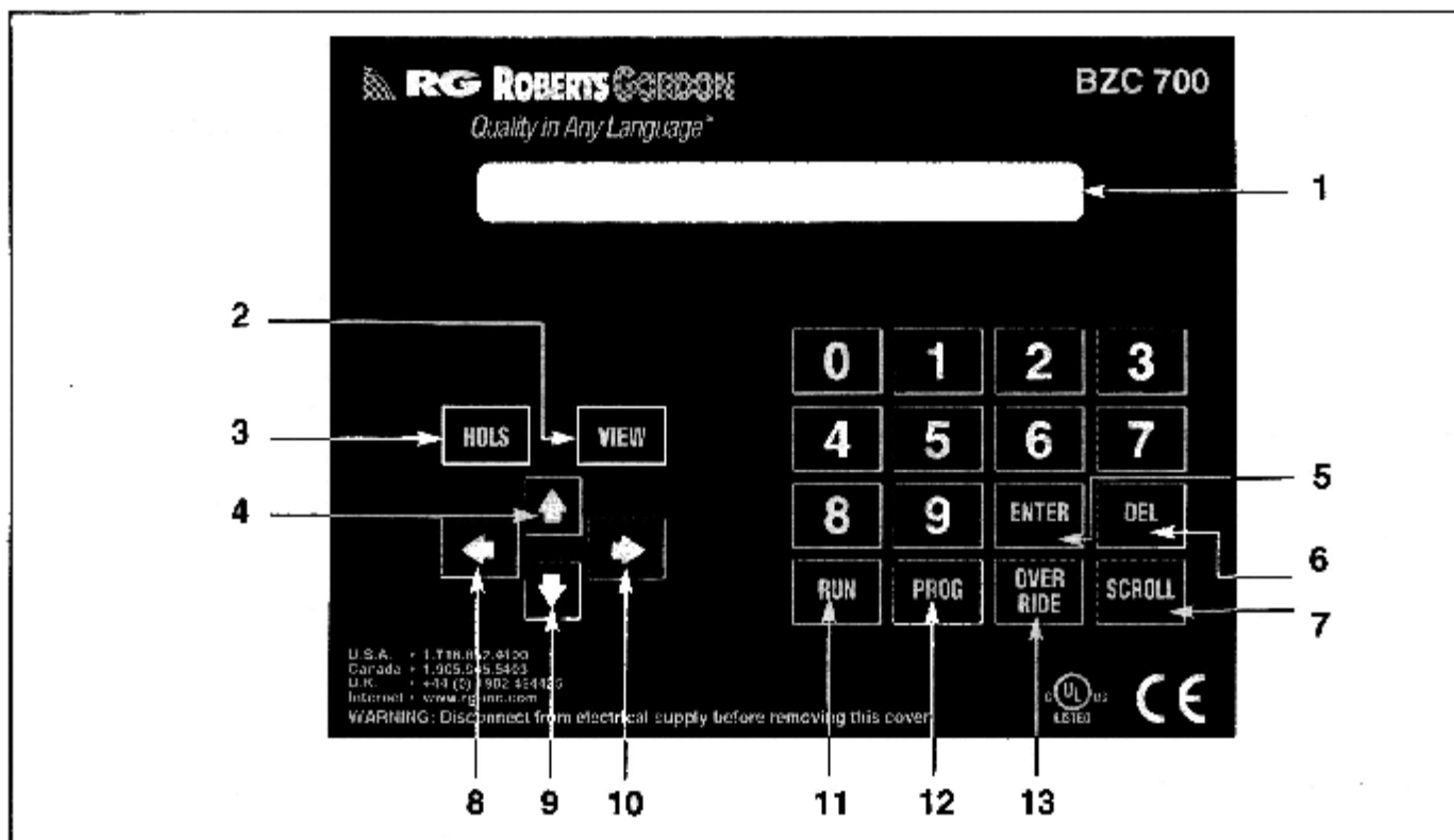
РИСУНОК 5 Кнопочная панель
