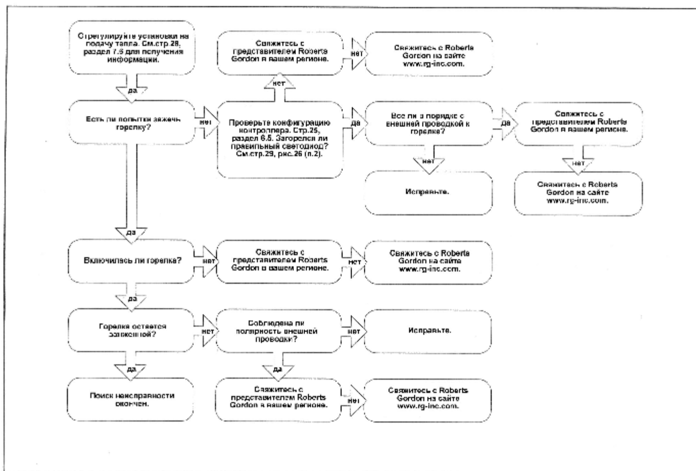
РИСУНОК 24 Поиск неисправности для единичного обогревателя
