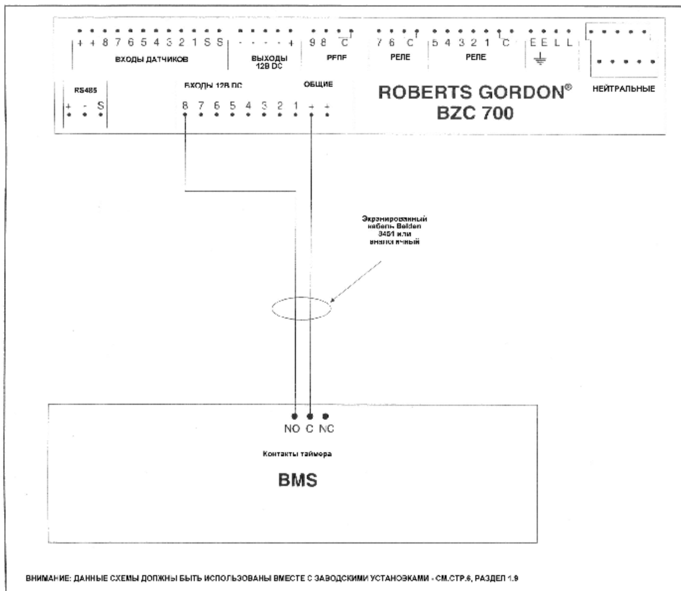
РИСУНОК 20 Типичная монтажная схема подключения к таймеру
