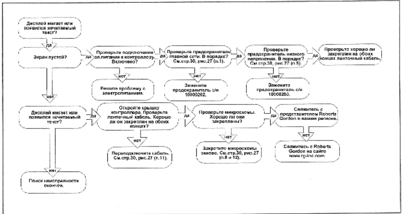
РИСУНОК 22 Поиск неисправности дисплея
