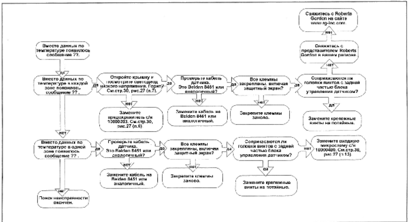
РИСУНОК 23 Поиск неисправности датчика
