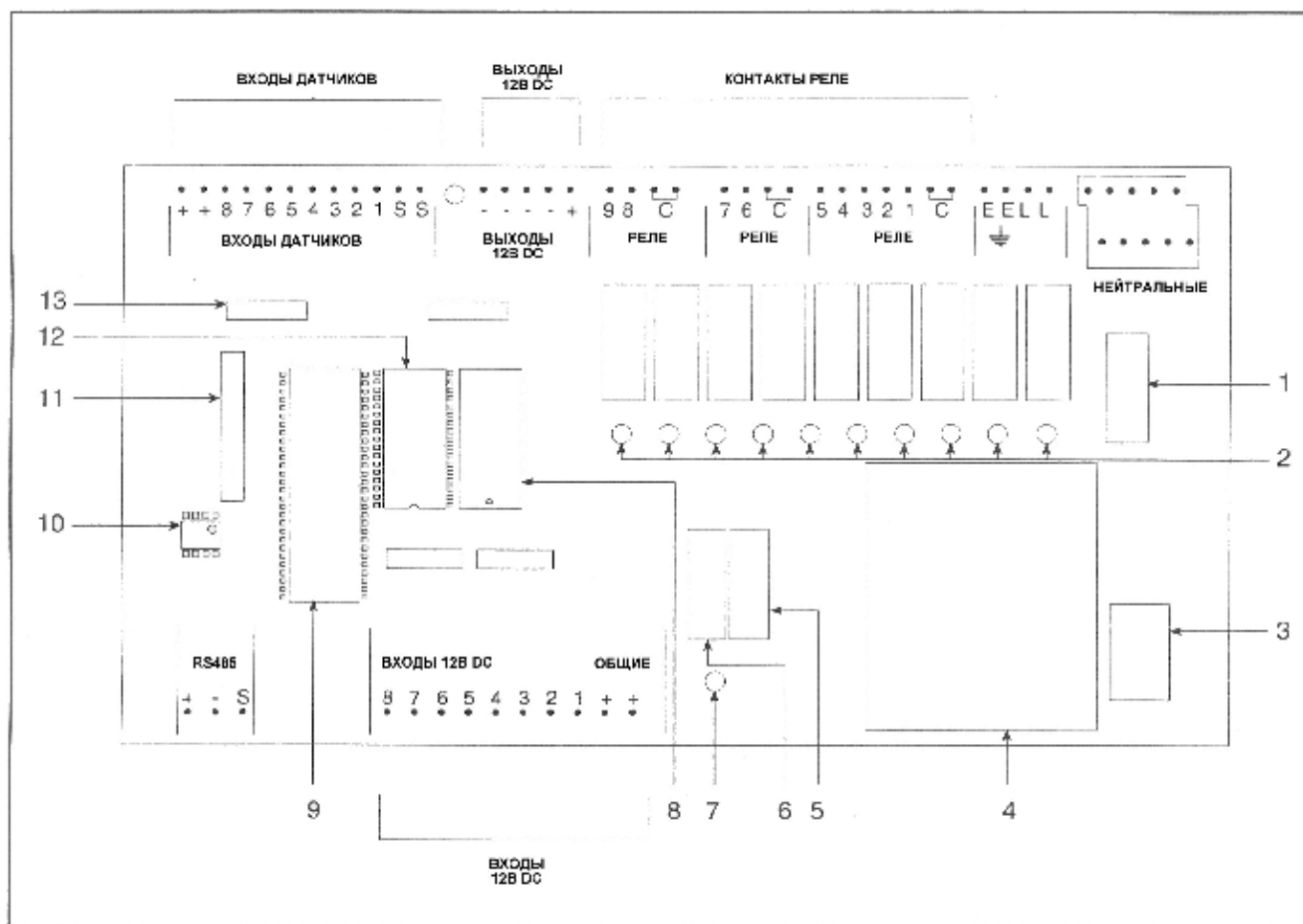
РИСУНОК 26 Внутренние компоненты Roberts Gordon® BZC 700
