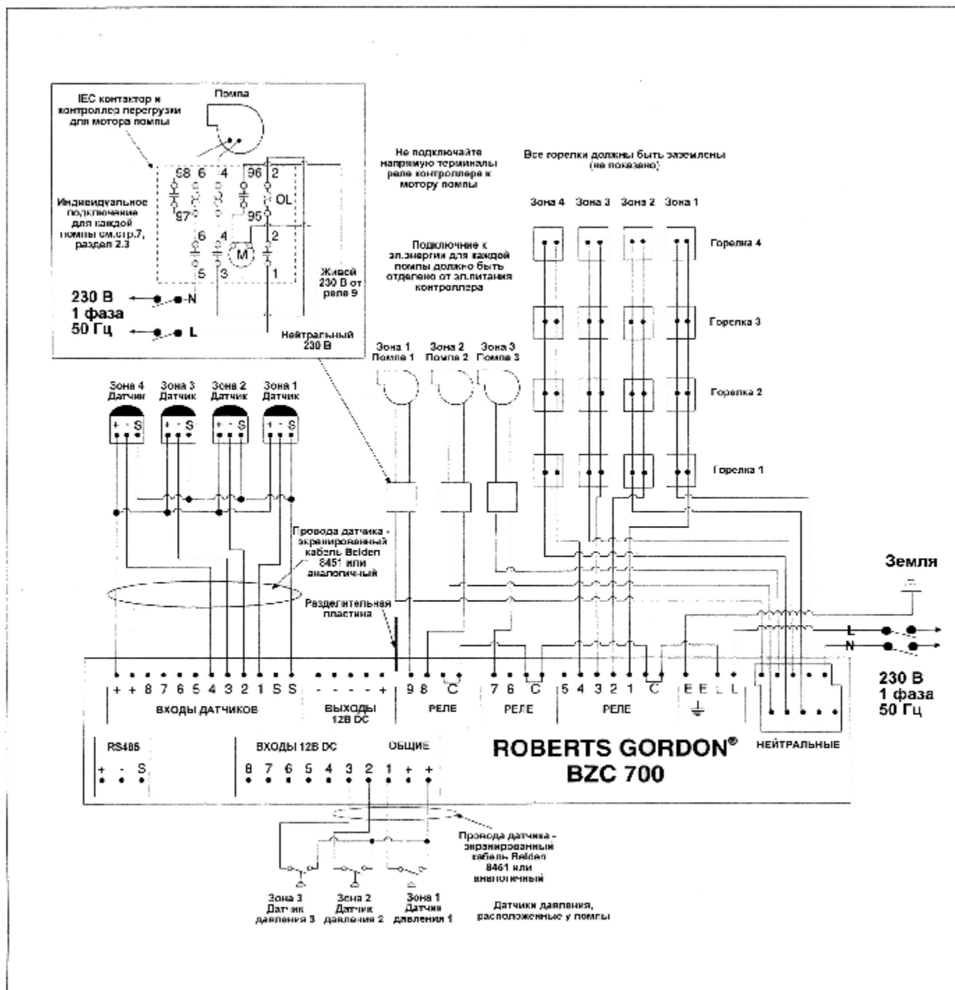
РИСУНОК 4 Пример схемы внешней электропроводки
