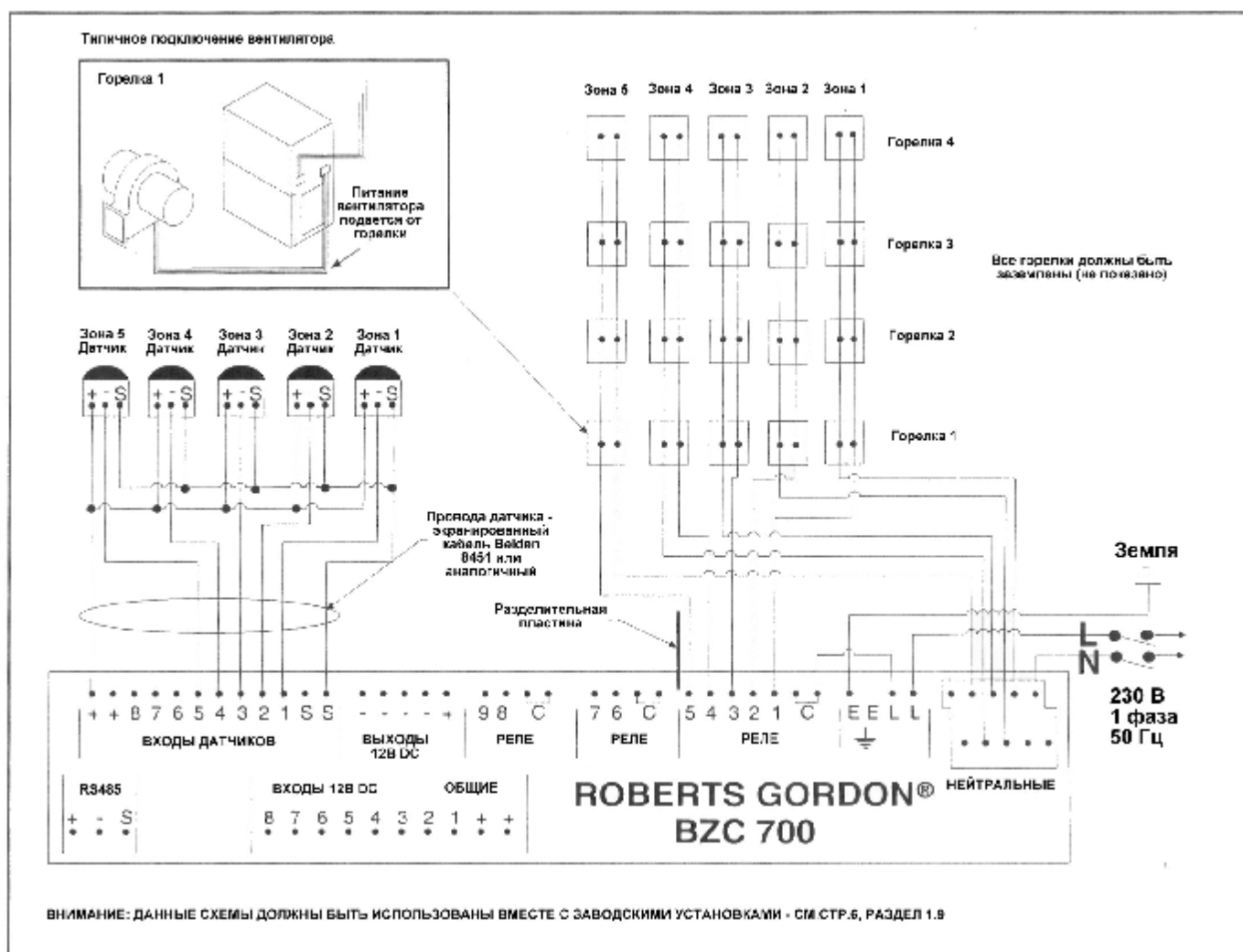
РИСУНОК 13 Типичная схема внешней проводки для единичных обогревателей серии BLACKHEAT® и CARIBE®
