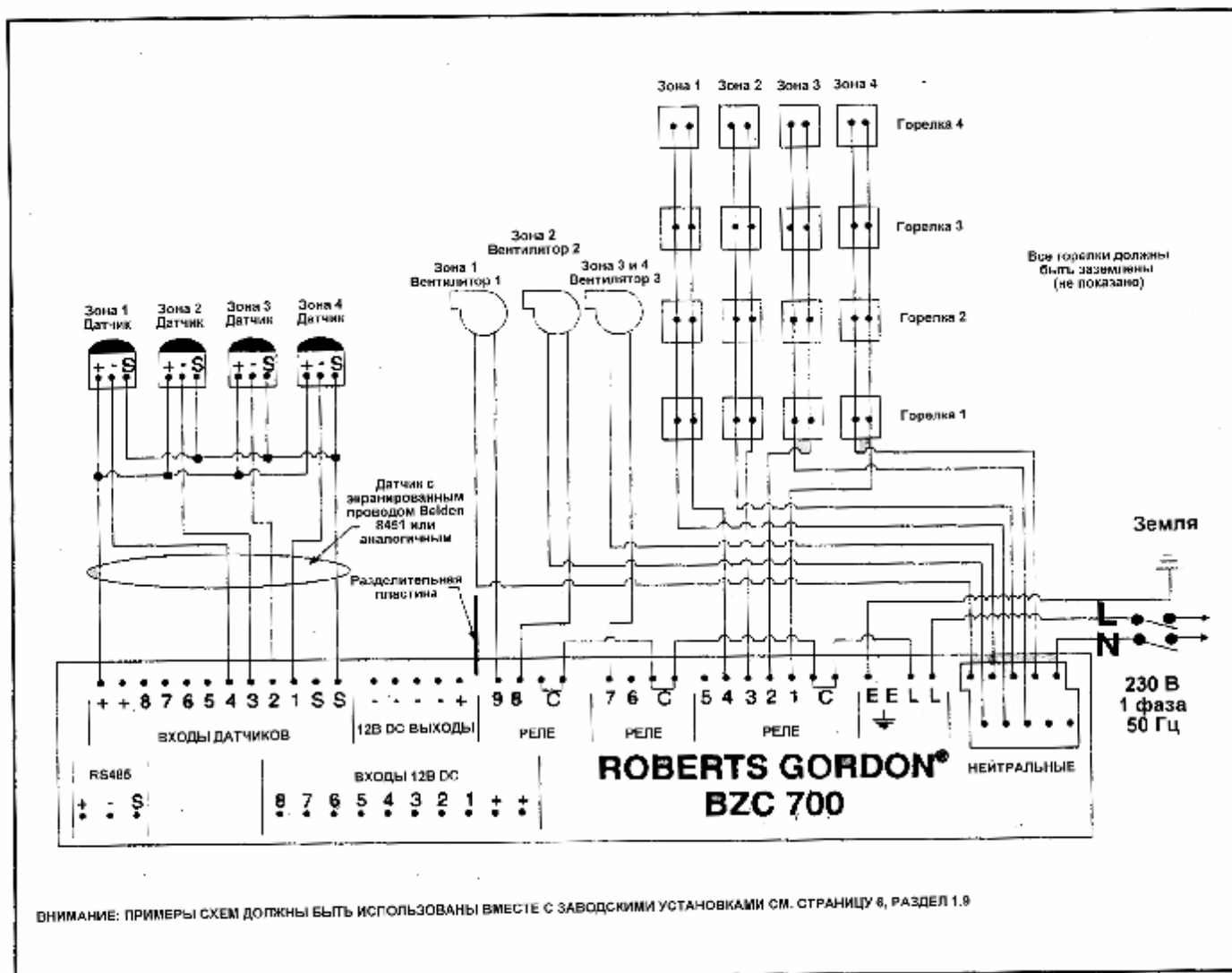
РИСУНОК 14 Типичная схема внешней проводки для системы обогревателей BLACKHEAT®.
