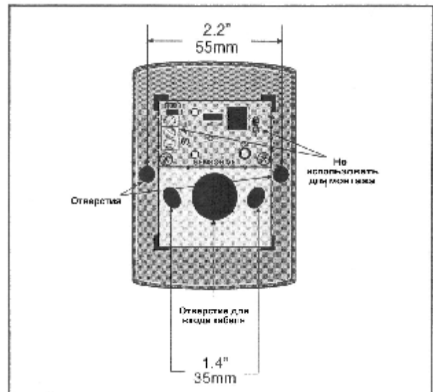
РИСУНОК 12 Элементы крепления
