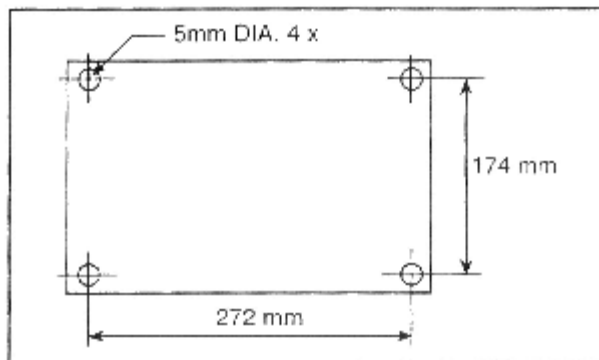
РИСУНОК 7. Расположение монтажных отверстий
