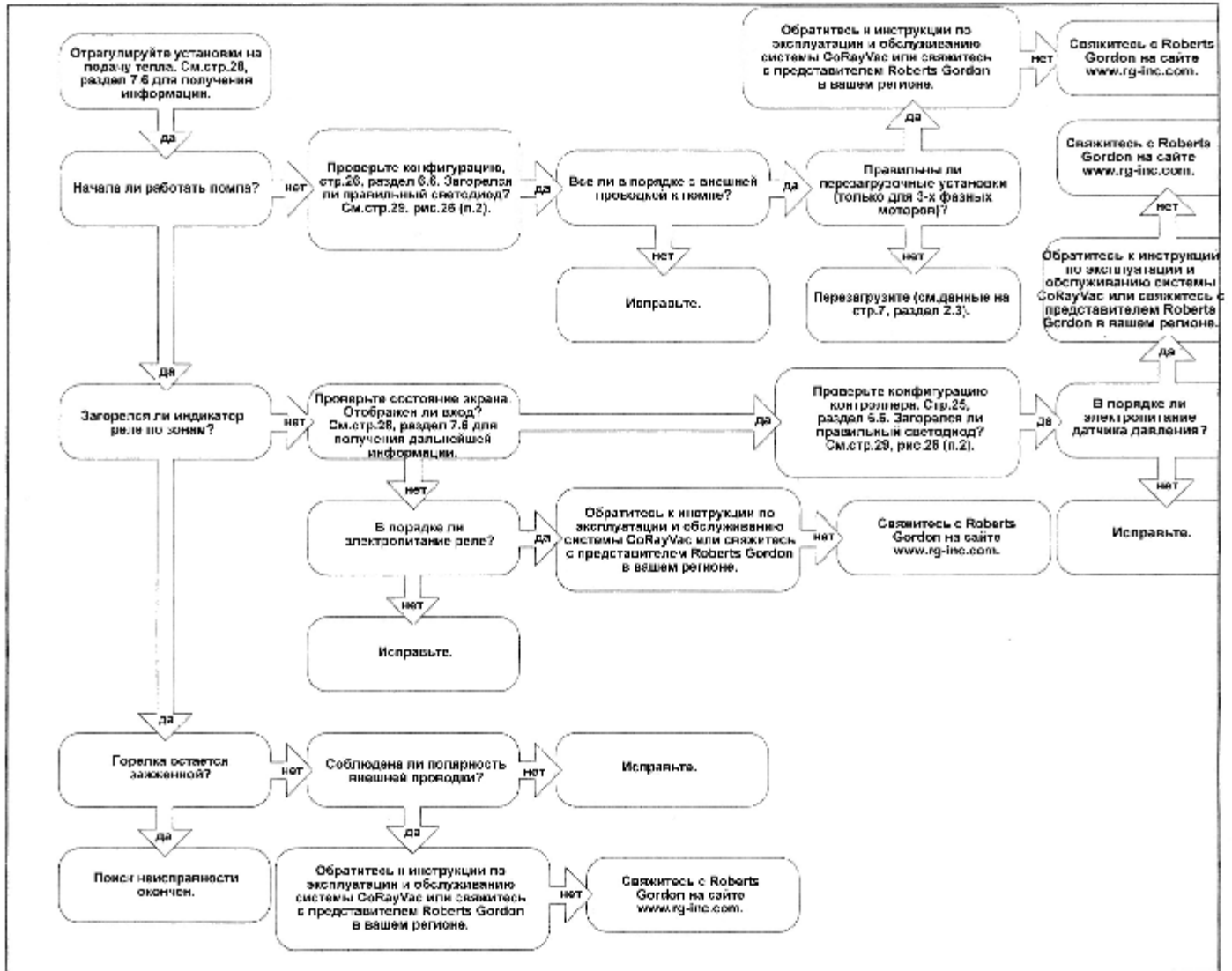
РИСУНОК 25 Поиск неисправности для CORAYVAC®
