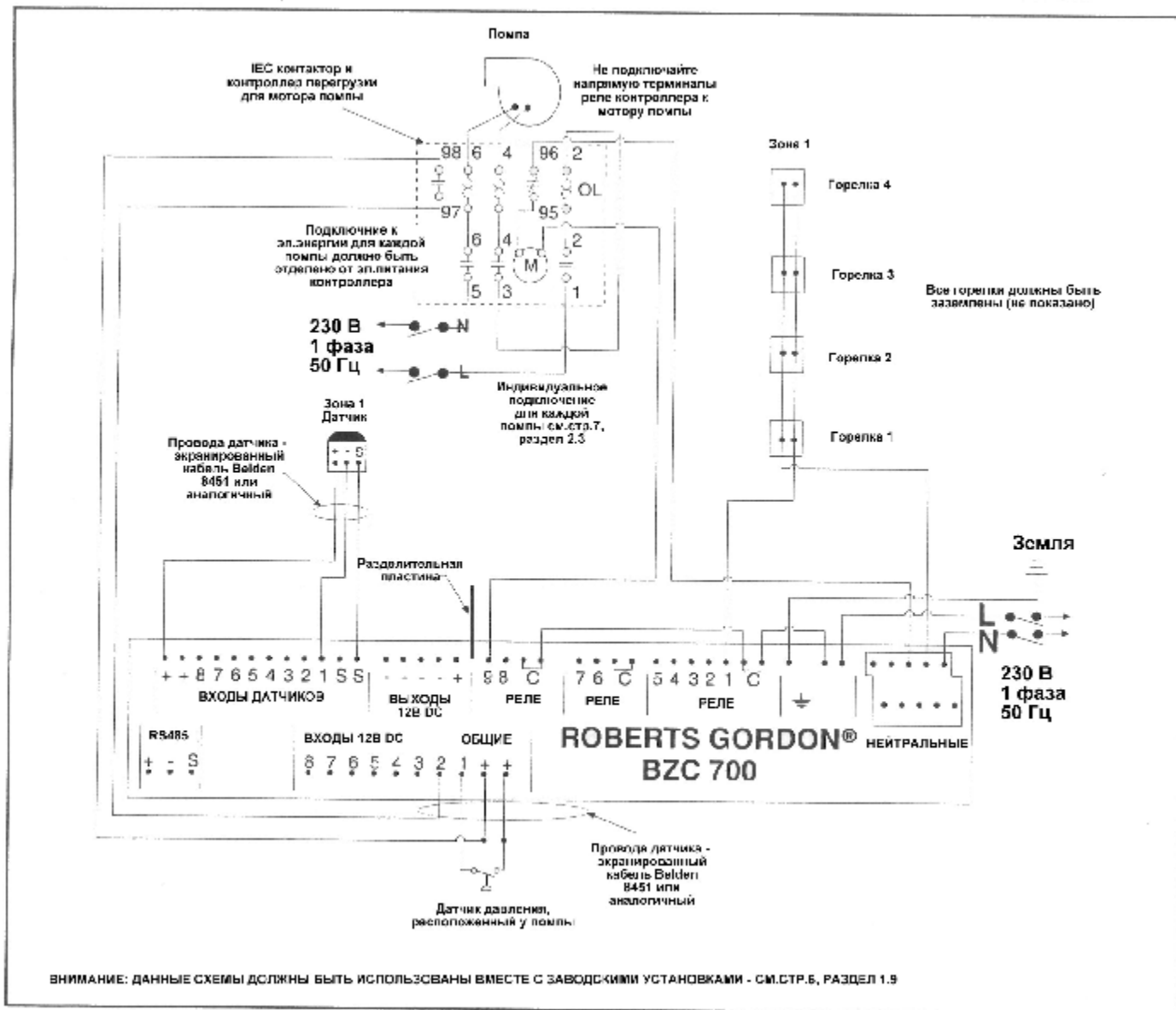
РИСУНОК 18 Типичная схема индикации отключения однофазной помпы
