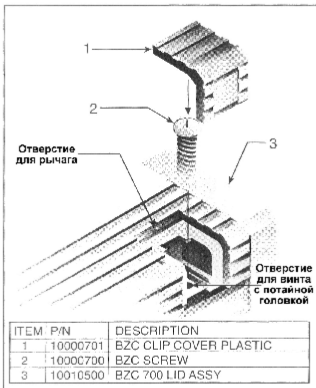
Рисунок 6. Деталь крышки контроллера Roberts Gordon® BZC 700
