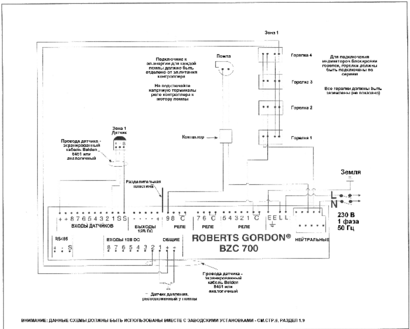
РИСУНОК 19 Типичная схема индикации блокировки горелки
