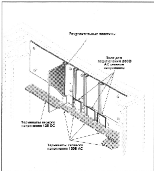
РИСУНОК 9. Детали разделительных пластин 3.2.11 Подсоедините заново резиновый кабель к блоку управления и верните на место крышку контроллера. Закрепите крышку винтами.
